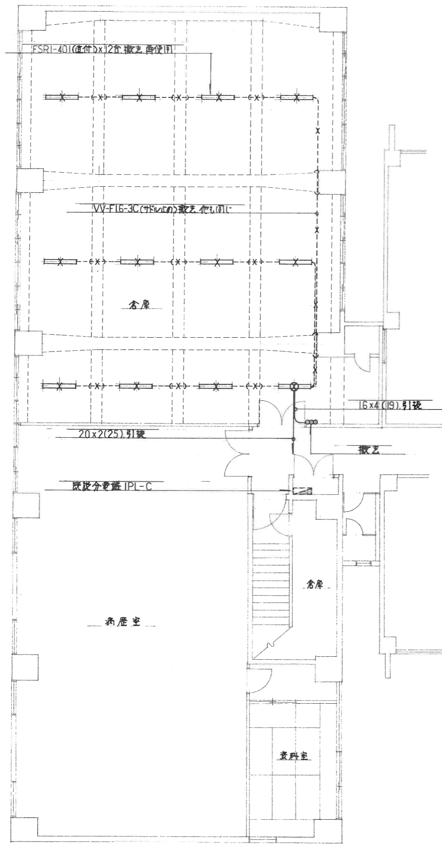
1F 改修前 1:100
