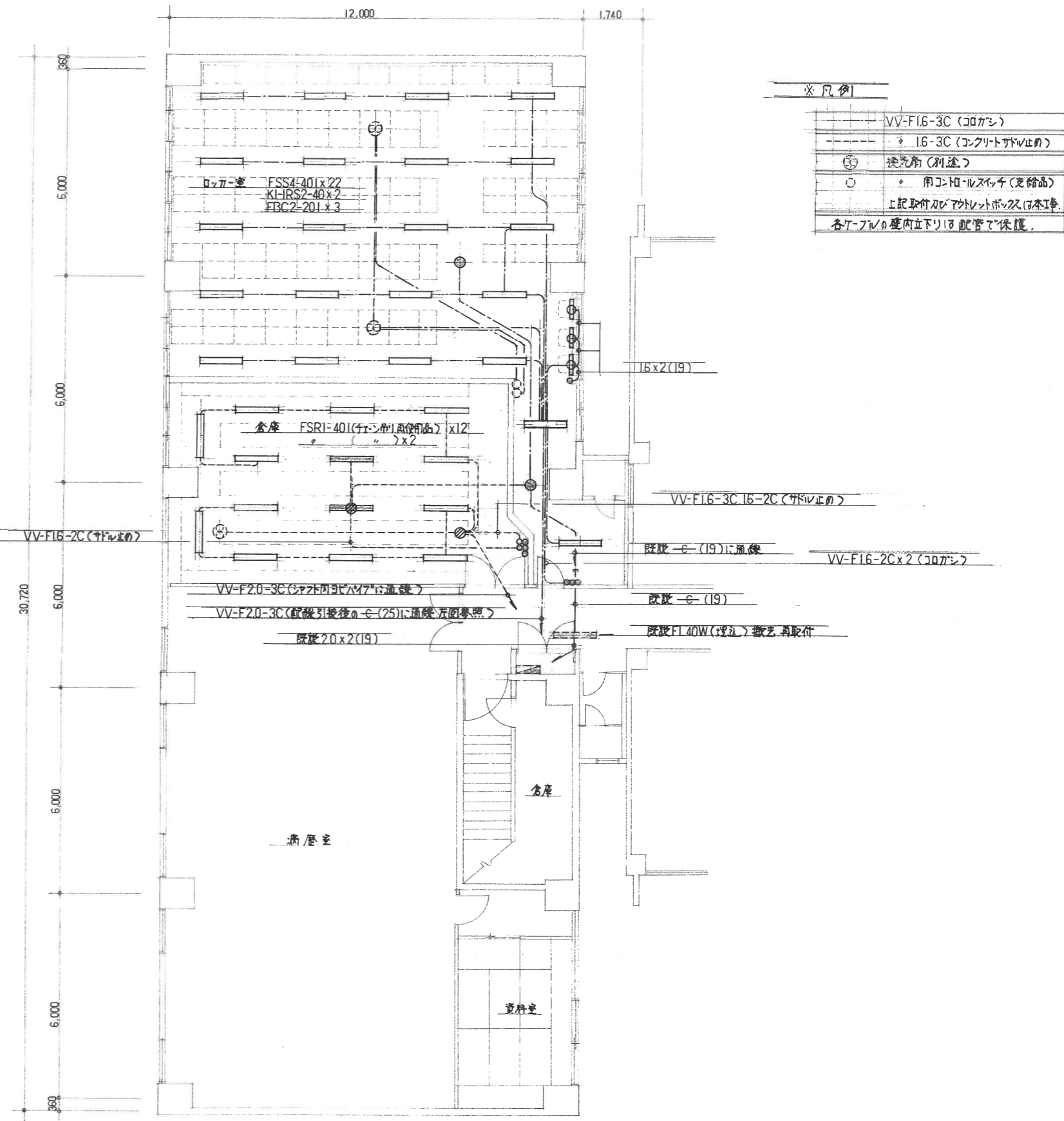
1F 改修後 1:100
