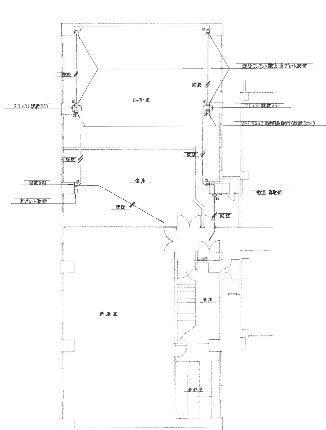
IF 改修後 1/100
